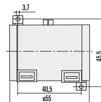
FISSAGGIO FIXING (mm)
