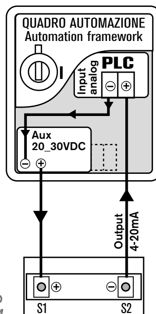
SCHEMA DI COLLEGAMENTO WIRING DIAGRAM
