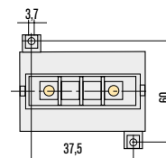
FISSAGGIO / FIXING (mm)
