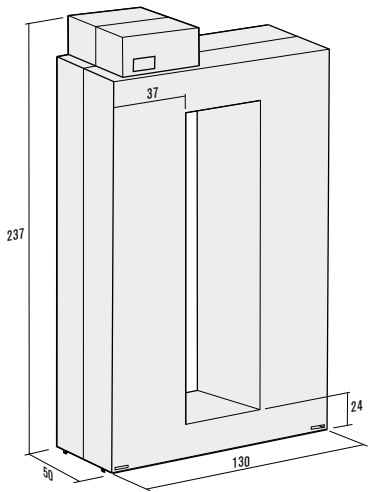
DIMENSIONI DIMENSIONS (mm)
