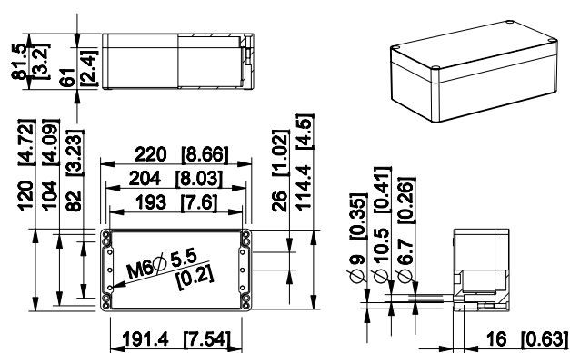
Ensto Cubo H 120 x 220 x 81,5 mm
