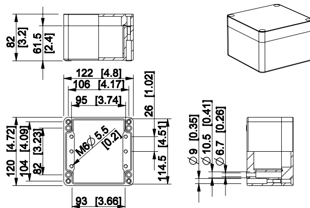
Ensto Cubo H 120 x 122 x 82 mm
