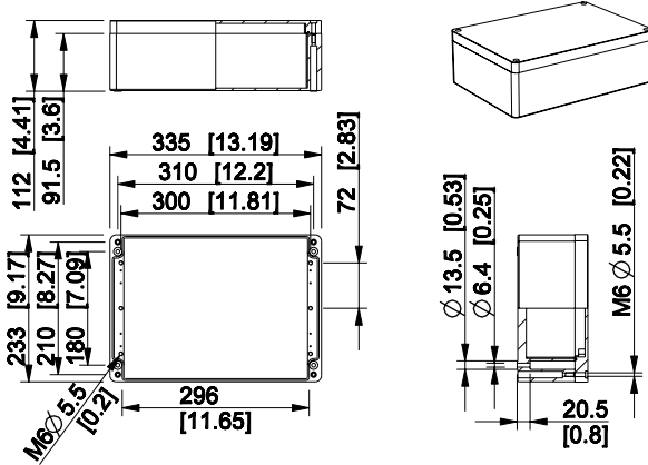
Ensto Cubo H 233 x 335 x 112 mm
