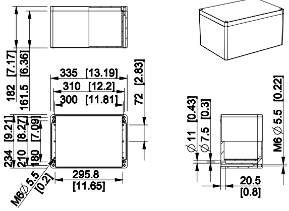
Ensto Cubo H 234 x 335 x 182 mm
