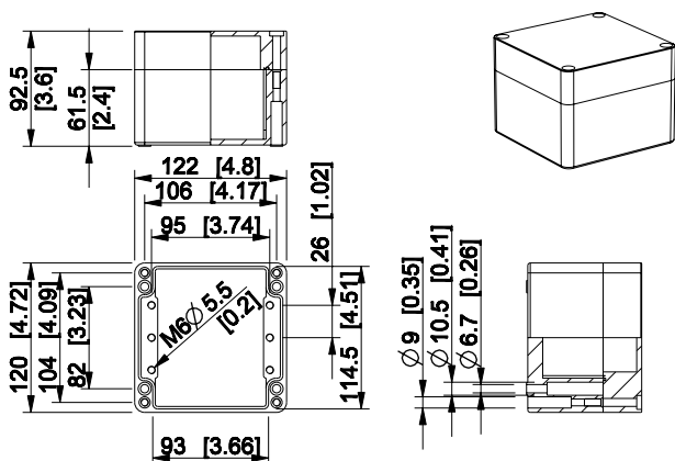
Ensto Cubo H 120 x 122 x 92,5 mm
