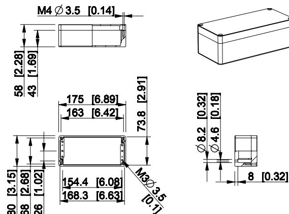
Ensto Cubo H 80 x 175 x 58 mm
