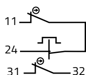
Elemento di contatto con automonitoraggio Contact block with self-monitoring
