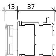
Elemento di contatto con automonitoraggio Contact block with self-monitoring
