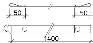
Cavo Spiralato / Spiral cable 12x0,5 mm 2
