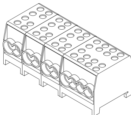
Isometrisch
