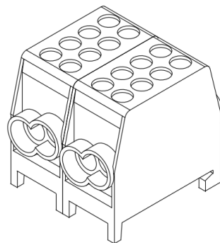
Isometrisch
