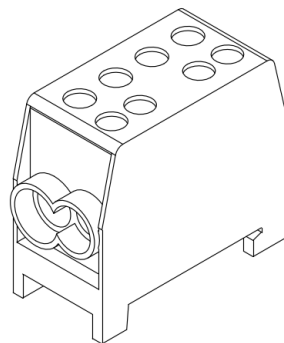
Isometrisch
